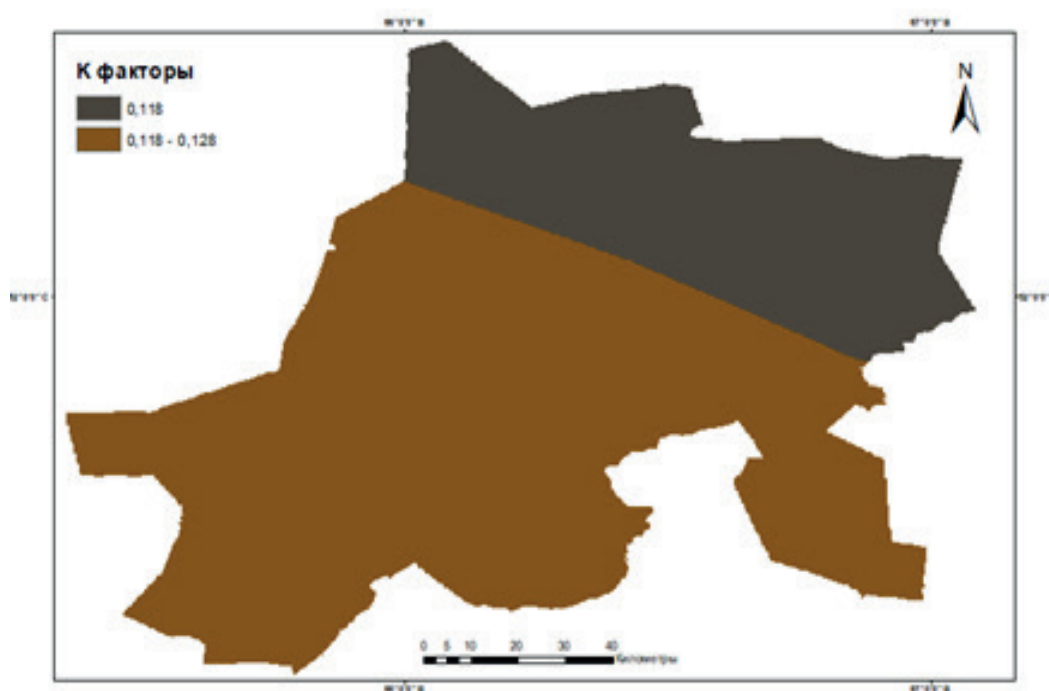
3-сурет – Ақмола облысы Есіл ауданының топырақ эрозиясының таралу коэффициенті
