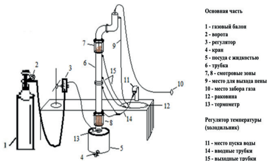
Рисунок 3 – Установка поглощения углекислого газа (CO 2 ) удобрением «Казуглеумус»
