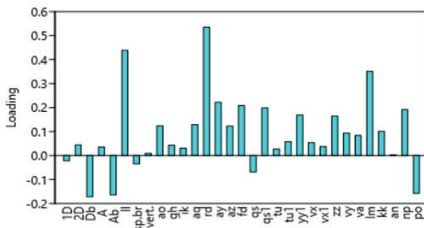
6-сурет – Бірінші басты компоненттер талдауы
