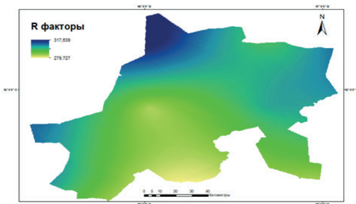
2-сурет – Ақмола облысы Есіл ауданының жауын-шашынның эрозиялық белсенділігінің таралуы
