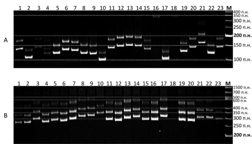
Рисунок 4. Электрофоретические профили продуктов ПЦР 23 родительских генотипов нута с использованием полиморфных STMS-маркеров: А – TA194; В – TA96. Обозначения дорожек:
