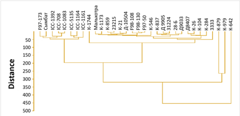
Рисунок 5. Дендрограмма генетического разнообразия 33 образцов нута по данным 5 STMS-маркеров
