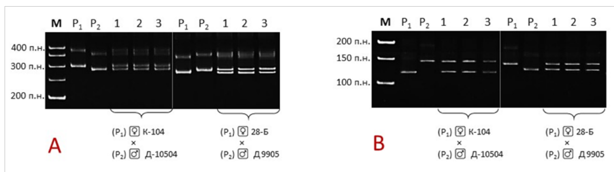
Рисунок 6. Результаты молекулярной верификации гибридов F1 с использованием STMS-маркеров TA194 (А) и TA96 (В) для комбинаций скрещиваний ♀ К-104 × ♂ Д-10504 и ♀ 28-Б × ♂ Д-9905; (Обозначения: М – ДНК-маркер молекулярных масс Step50 Plus (Биолабмикс, Россия); P1 – материнская форма; P2 – отцовская форма; 1, 2, 3 – анализируемые гибридные растения F1)
